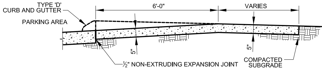
SECTION A-A
